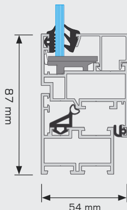
przekrój okna
