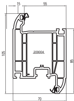
100008 - (DS85WF) INWARD OPENING DOOR SASH
