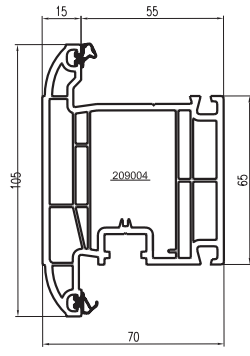
100009 - (DS105WF) OUTWARD OPENING DOOR SASH
