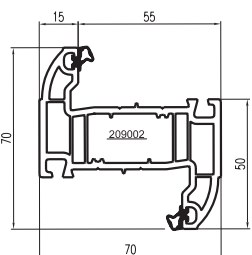
100012 - (ZM70WF) SLIM 'Z' TRANSOM/MULLION
